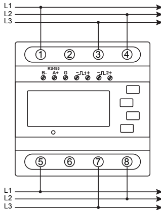
Réseau TRI sans neutre
